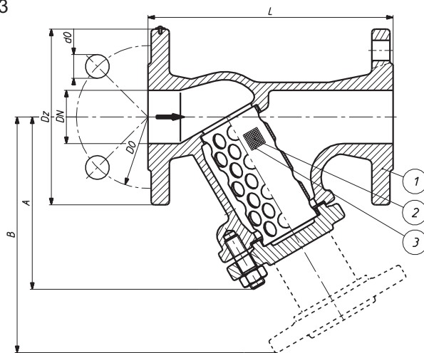
Rys. 1 Budowa i wymiary filtra
