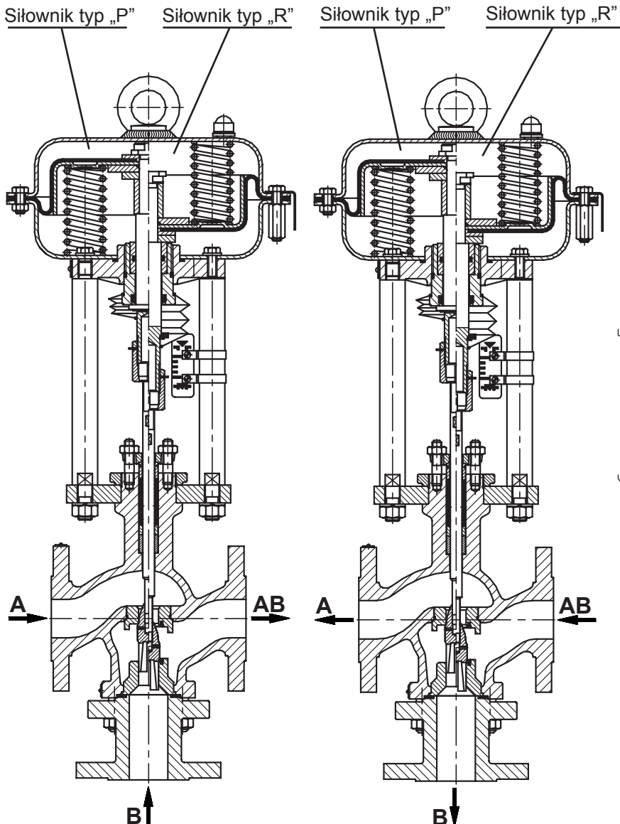
Rys.5. P/R-Z3M - Mieszający
