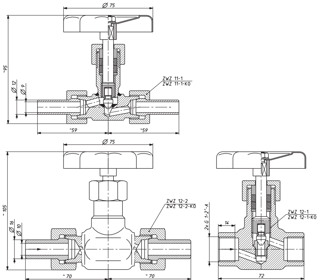
Budowa i wymiary zaworów Rodzaje wykonania zaworu zaporowego
