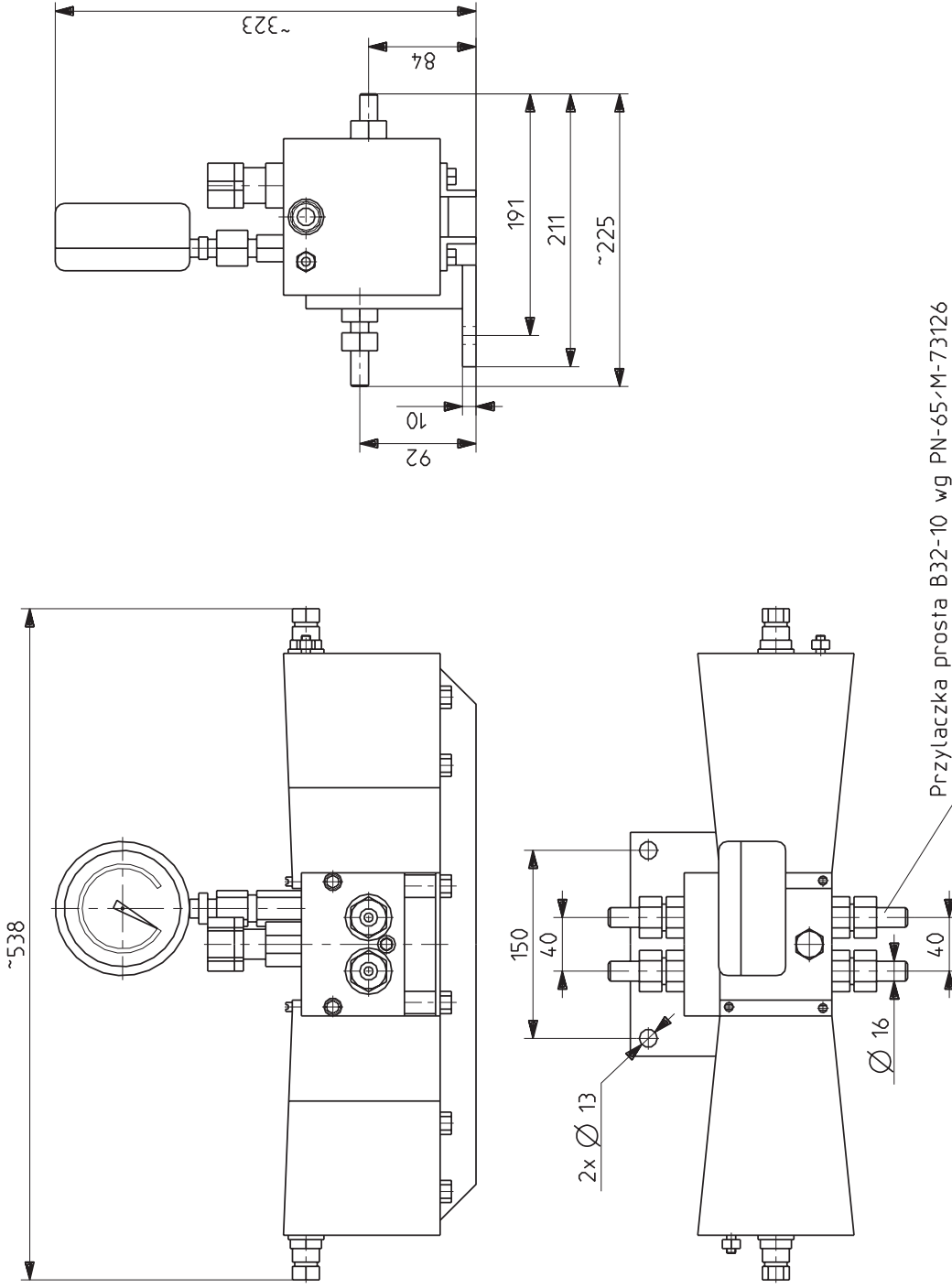
Rys.2 Wymiary zewnętrzne i przyłączeniowe rozdzielacza ER
