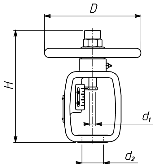
Rysunek 10. Napęd ręczny typ 20.
