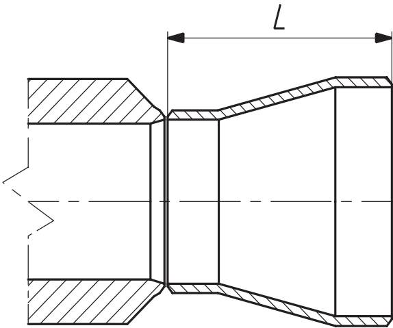
Rysunek 7. Króciec redukcyjny
