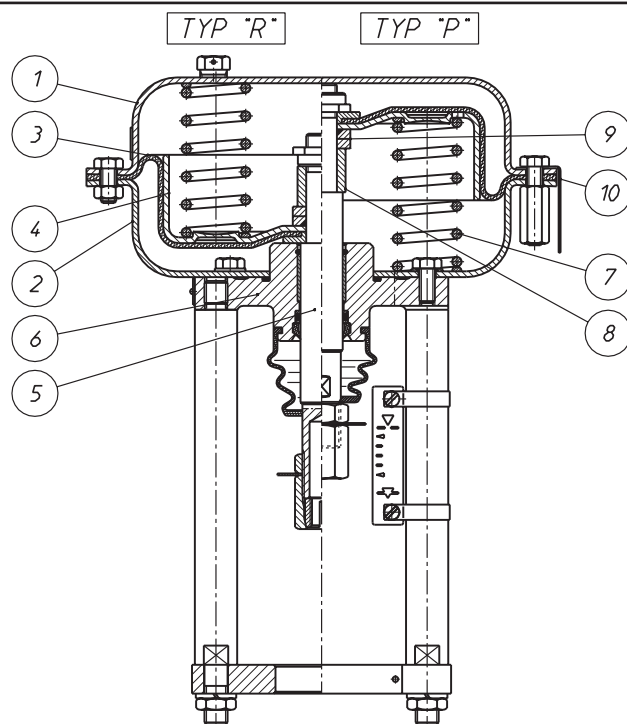
Rysunek 5. Siłownik wielosprężynowy typ P/R
